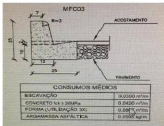
Figura 1. Perfil do meio fio MFC 03.
