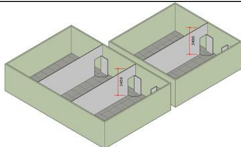
Perspectiva – Escala 1/100
