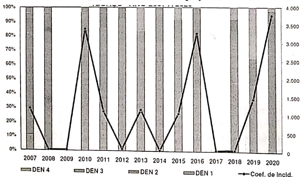
Gráfico 1 – Sorotipos circulantes, Foz do Iguaçu – 2007 e 2020.
